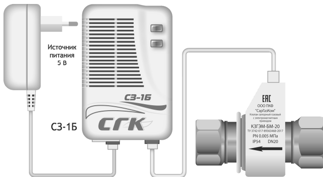
Рис. А1. Сигнализаторы загазованности бытовые СЗ-Б с клапаном типа КЗЭМ-БМ.
