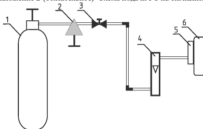
Рисунок Б.1 – Рекомендуемая схема подачи ГС на вход сигнал. загазованности бытовых СЗ-Б 1 – источник ГС (баллон или ГГС-03-03); 2 – редуктор с вентилем точной регулировки (при использовании ГС в баллонах под давлением); 3 – вентиль точной регулировки (при использовании ГС в баллонах под давлением); 4 – индикатор расхода (ротаметр); 5 – насадка для подачи ГС; 6 – сигнализатор;
