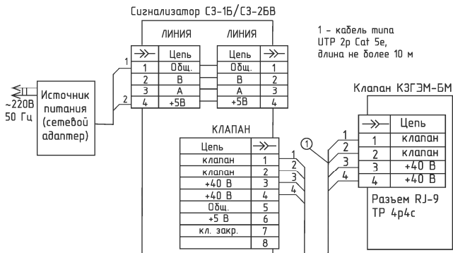
Рис. А2. Схема электрических соединений сигнализаторов СЗ-Б и бытового электромагнитного клапана КЗЭМ-Б(без узла индикации положения клапана).
