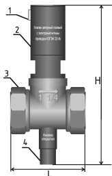
Рисунок 3. – Клапан КЗГЭМ-Б.
